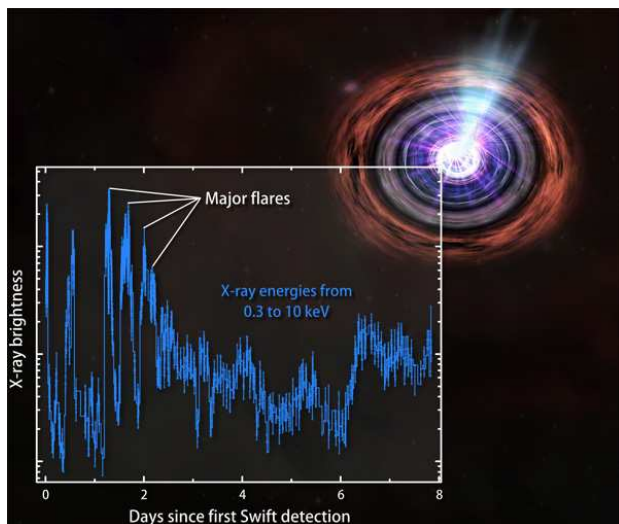
Рис. 2. Колебания интенсивности всплеска GRB 110328A после его обнаружения. График из пресс-релиза НАСА: NASA/Swift/Penn State/J. Kennea с сайта http://elementy.ru . Однако ранее теоретики показали, что рождению джетов благоприятствуют магнитные поля именно с той конфигурацией, которая была смоделирована в новой работе.
